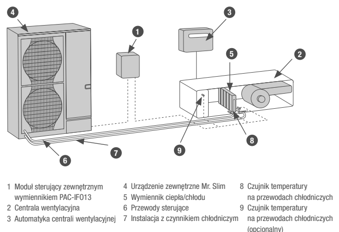
Zastosowanie modułu sterującego zewnętrznym wymiennikiem z instalacją wentylacyjną
